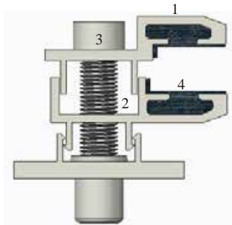
图 6 单边夹具示意图
