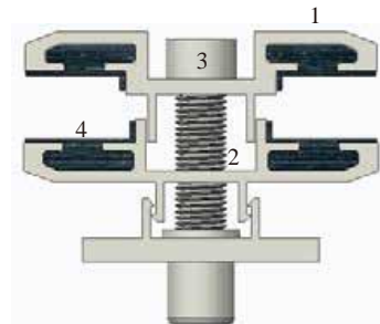
图 7 双边夹具示意图
