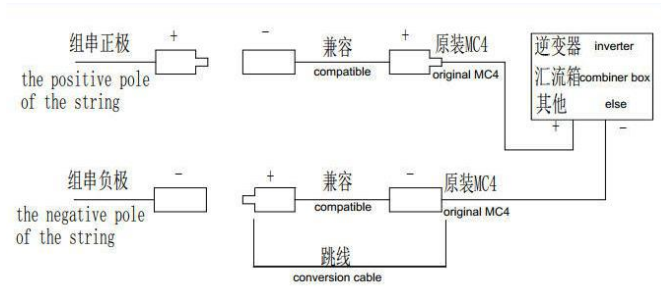
图 11 接线安装示意图
