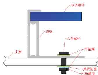
图 5 螺丝安装示意图
