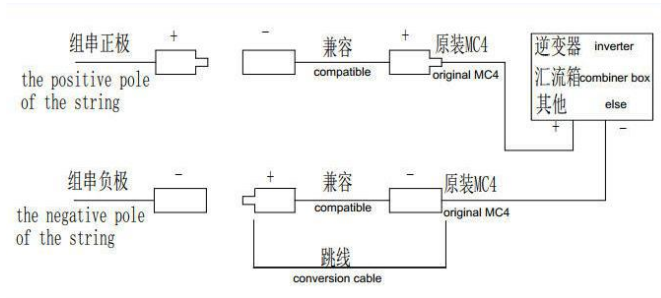
图9 接线安装示意图
